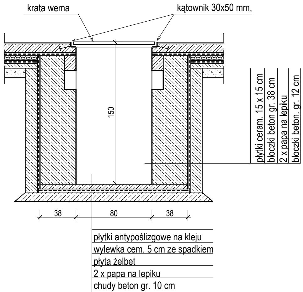
PRZEKRÓJ D - D 1:25
