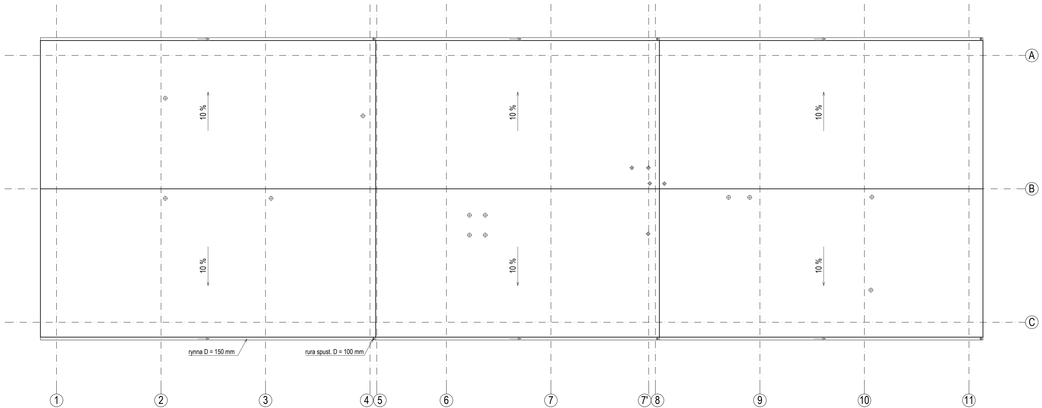
RZUT DACHU 1:100
