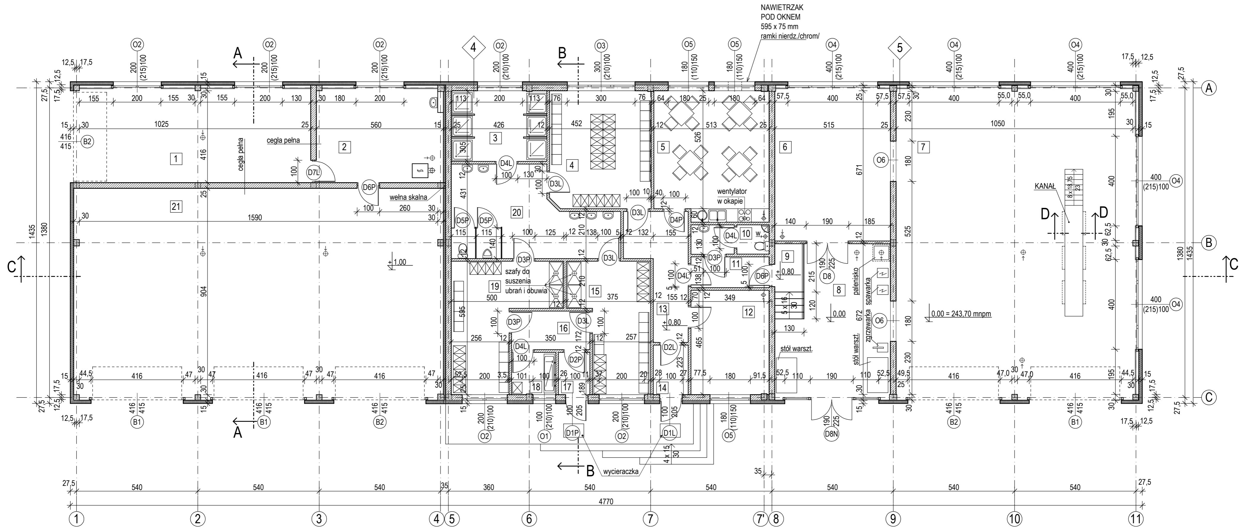
RZUT PARTERU 1:100
