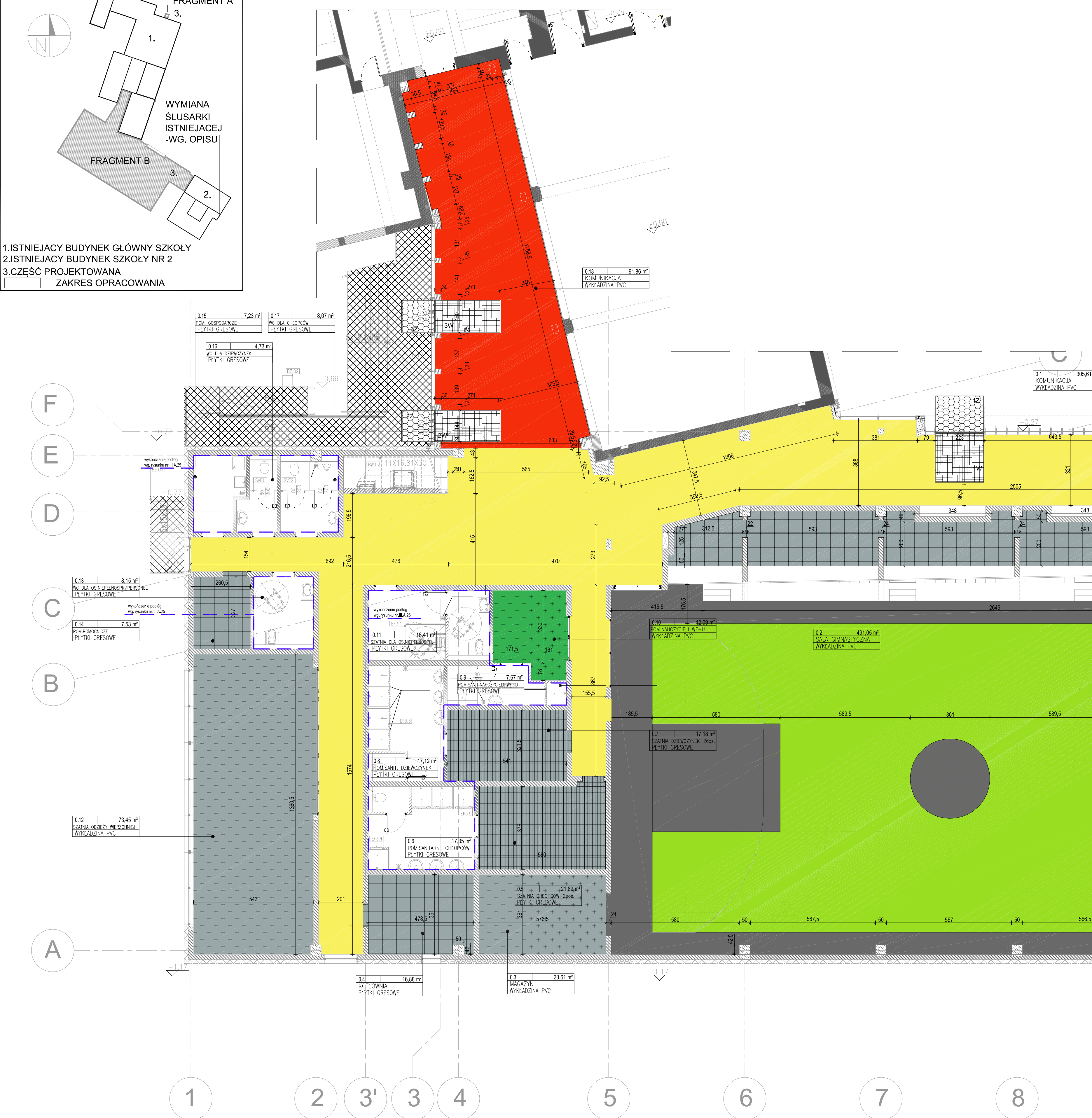
FRAGMENT B - RZUT PARTERU
