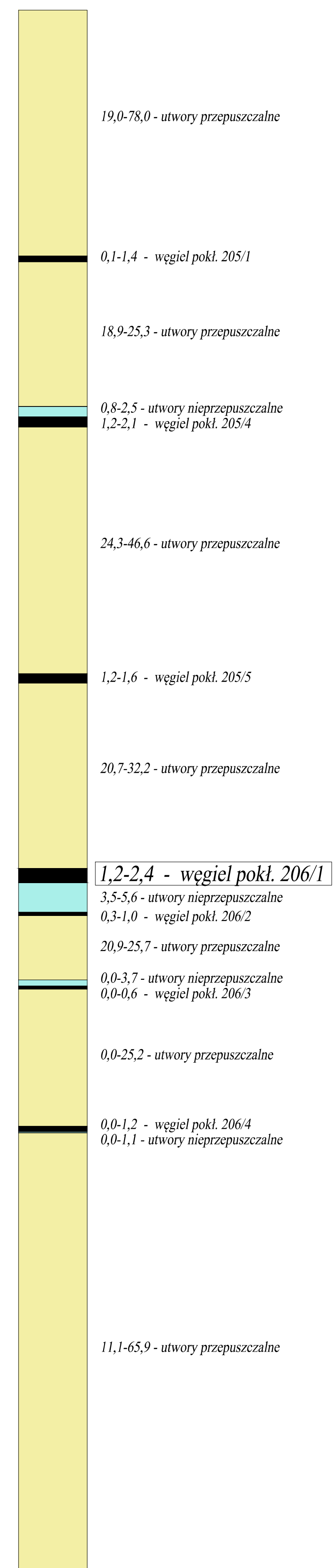
Profil hydrogeologiczny pokładu węgla 206/1
