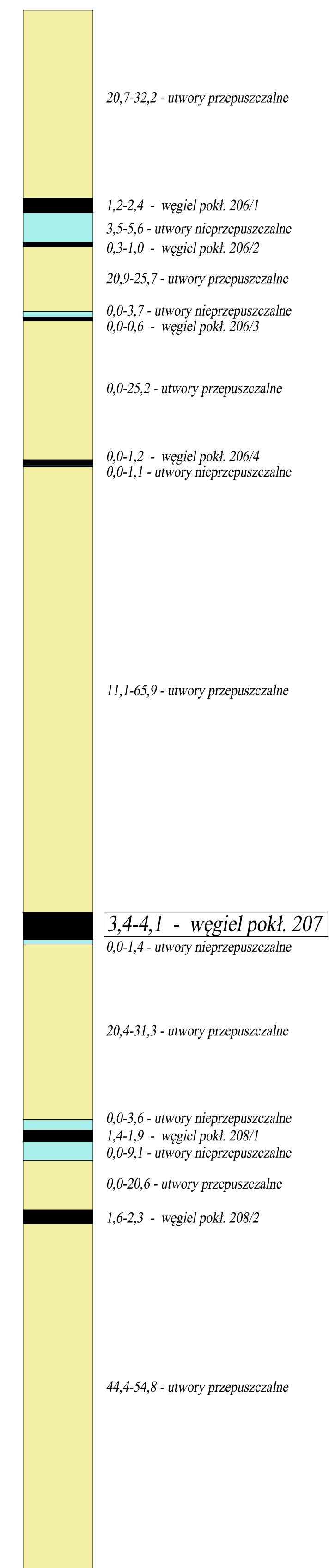
Profil hydrogeologiczny pokładu węgla 207
