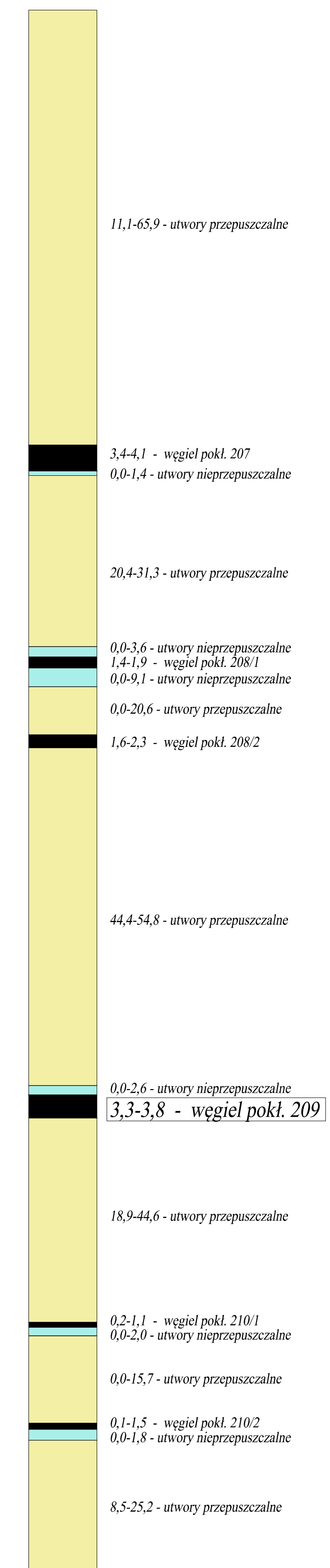
Profil hydrogeologiczny pokładu węgla 209
